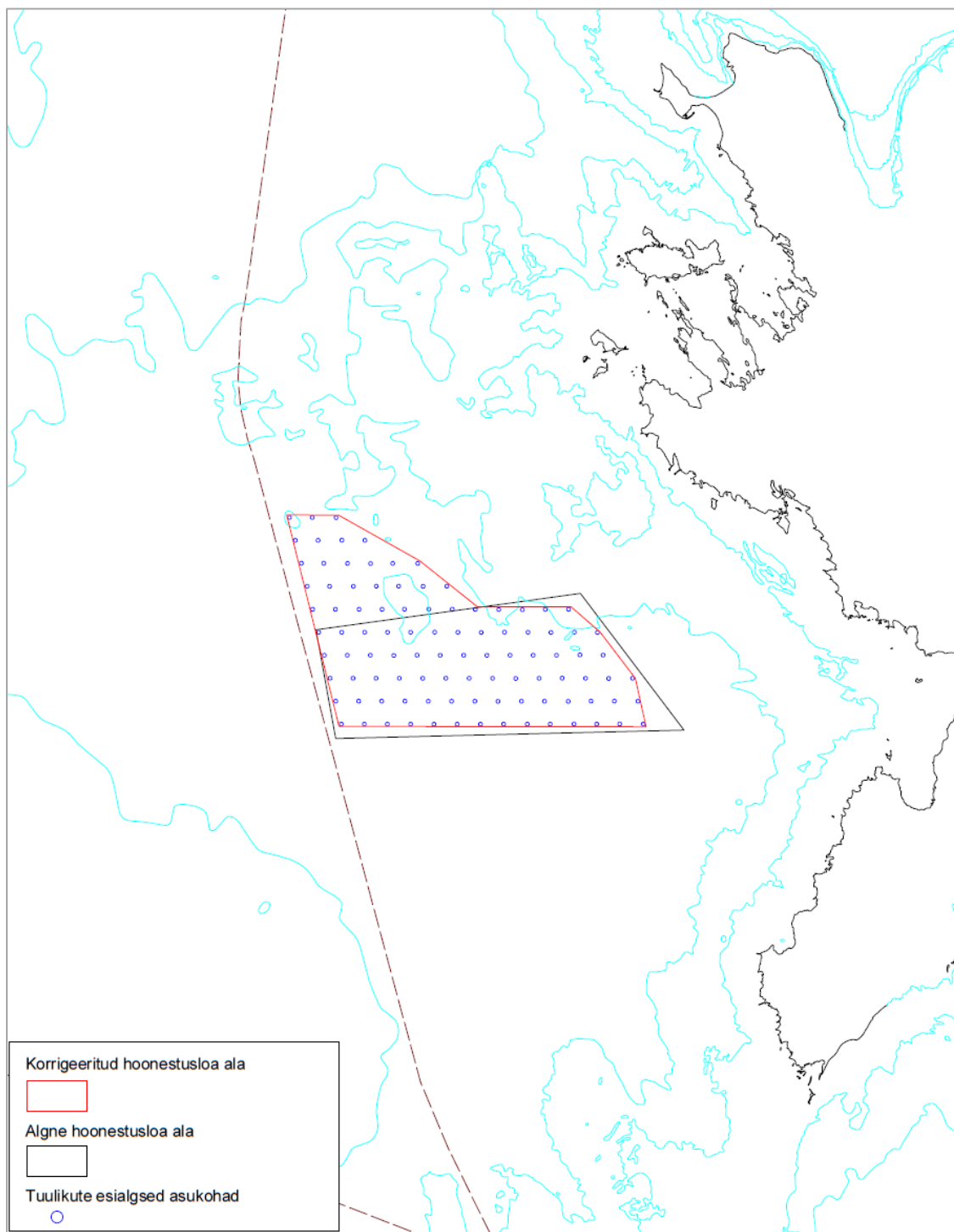
Joonis 1. Vabariigi Valitsuse 28.05.2020 korralduse nr 183 kohane ala ning taotletava hoonestusloa korrigeeritud ala, joonisel on esitatud ka elektrituulikute võimalikud asukohad.
